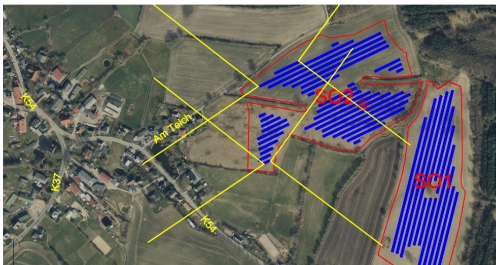
Abbildung 15: Bodennahen Reflexionsrichtungen des Gebiets SO2 in der Horizontalstellung der Trackersysteme als gelbe Winkel mit 300 m Schenkellänge, angetragen an ausgewählte Eckpunkte der belegten Fläche
