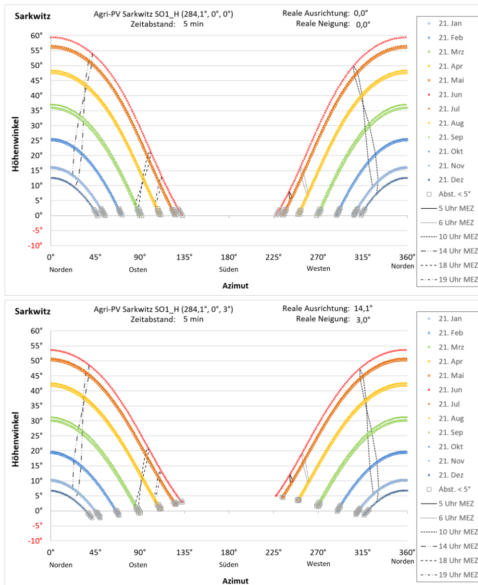
Abbildung 8: Reflexionsdiagramme für das Gebiet SO1 in Horizontalposition mit 0° und 3° Neigung der Drehachse
