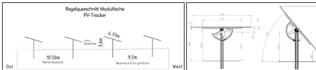
Abbildung 7: bemaßte Ansichten der Trackersysteme; Quelle: Kundenmaterial
