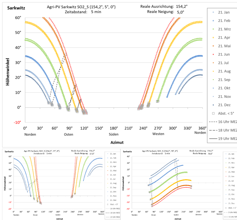
Abbildung 13: Reflexionsdiagramme für PV-Module des Gebiets SO2 bei Ausrichtung nach Süden mit einer Neigung von 5°, 17° und 70°
