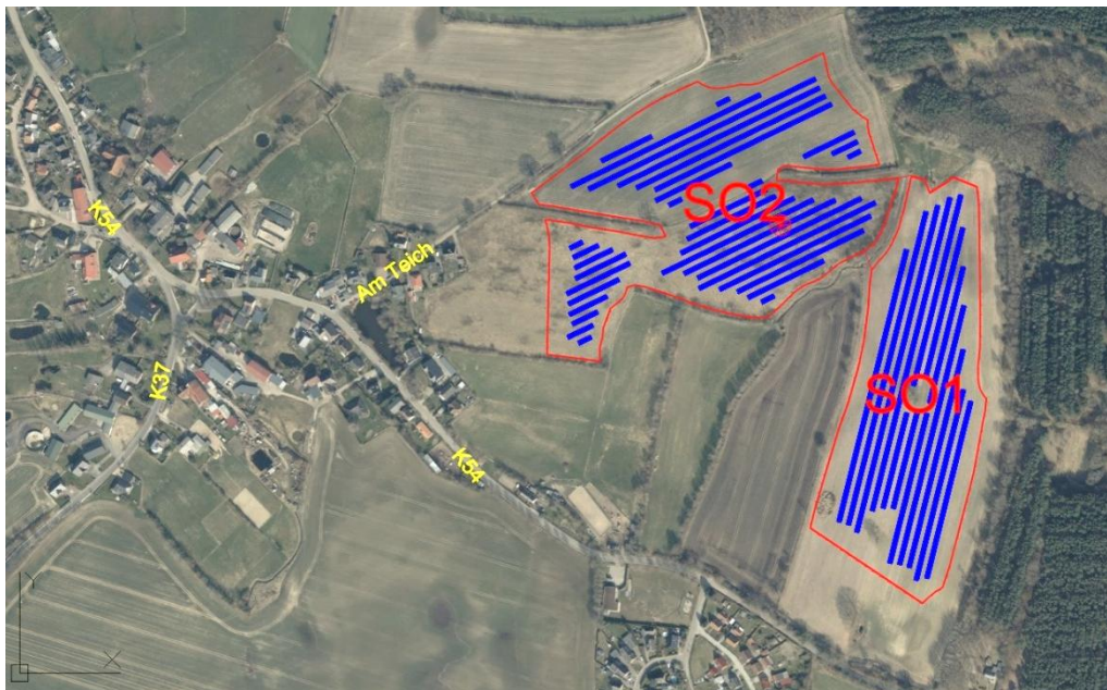
Abbildung 6: Belegungsplan der geplanten Agri-PV-Anlage, Stand Mai 2026
