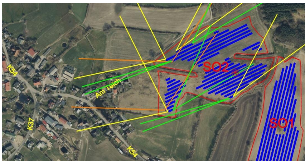
Abbildung 17: Bodennahen Reflexionsrichtungen des Gebiets SO2 bei Nordausrichtung der Trackersysteme durch gelbe (5° Neigung), orangene (17°) und grüne (70°) Winkel mit 300 m Schenkellänge, angetragen an ausgewählte Eckpunkte
