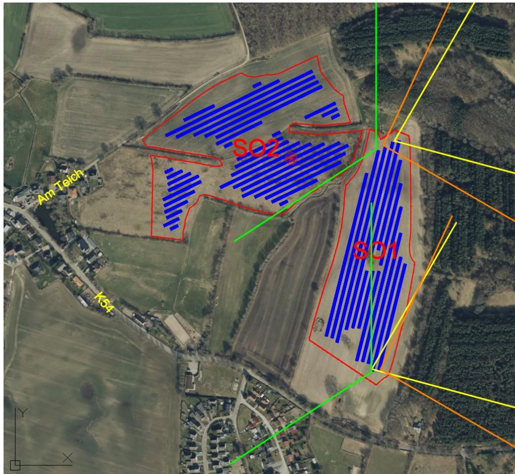
Abbildung 11: Darstellung der bodennahen Reflexionsrichtungen der PV-Module des Gebiets SO1 für Sonderpositionen der Trackersysteme durch gelbe (Horizontalposition), orangene (Ostausrichtung) und grüne (Westausrichtung) Winkel mit 300 m Schenkellänge, angetragenen an ausgewählte Eckpunkte der belegten Fläche
