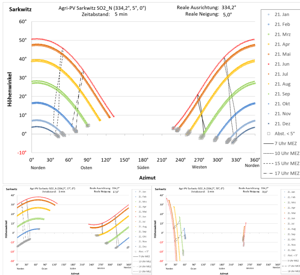
Abbildung 14: Reflexionsdiagramme für PV-Module des Gebiets SO2 bei Ausrichtung nach Norden mit einer Neigung von 5° (oben), 17° (unten links) und 70° (unten rechts)
