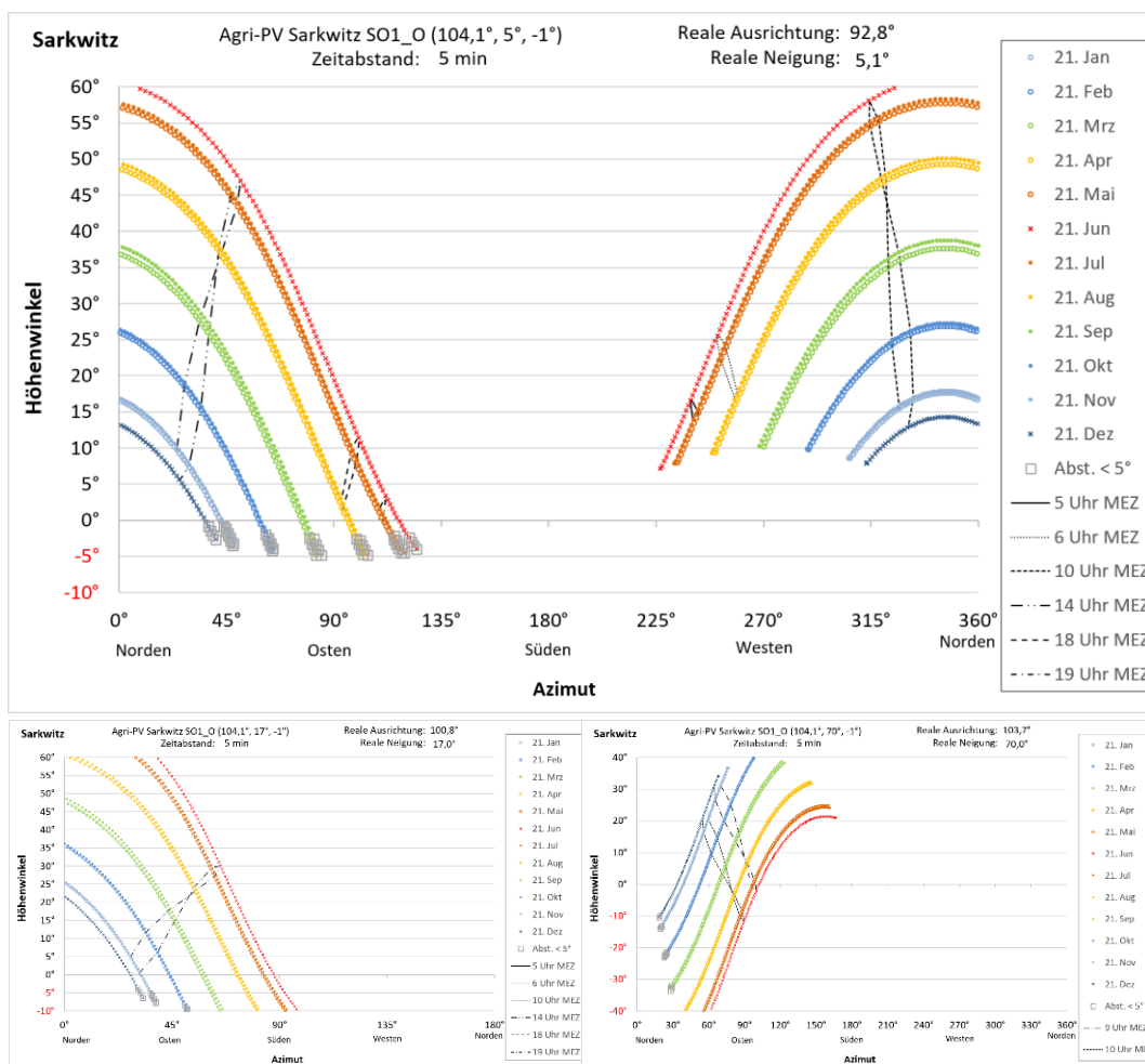
Abbildung 9: Reflexionsdiagramme für PV-Module des Gebiets SO1 bei Ausrichtung nach Osten mit einer Neigung von 5°, 17° und 70°
