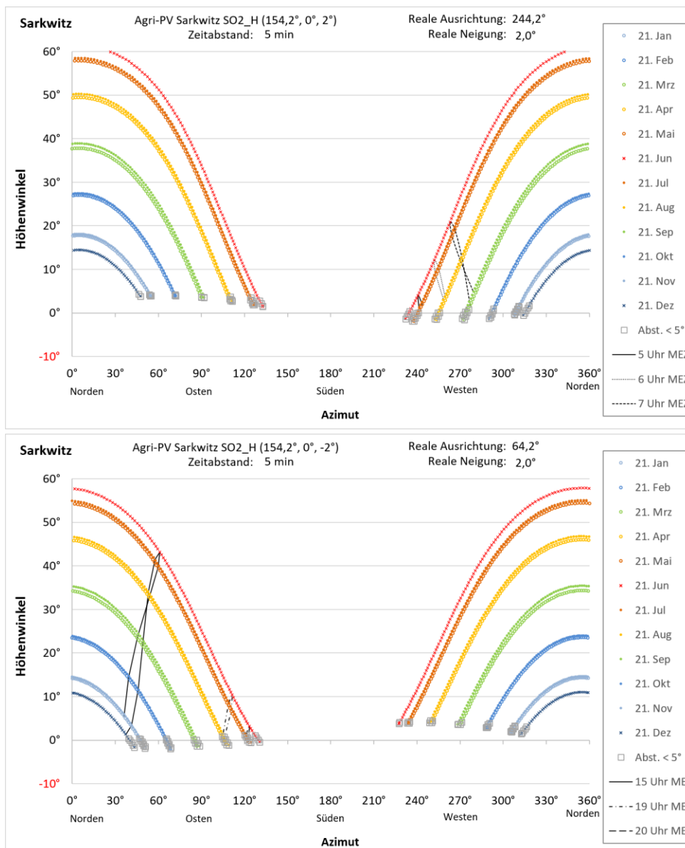
Abbildung 12: Reflexionsdiagramme für das Gebiet SO2 in Horizontalposition mit 2^\circ und -2^\circ Neigung der Drehachse
