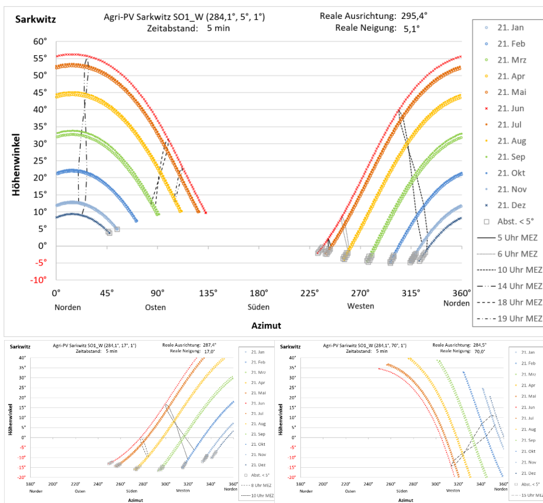
Abbildung 10: Reflexionsdiagramme für PV-Module des Gebiets SO1 bei Ausrichtung nach Westen mit einer Neigung von 5° (oben), 17° (unten links) und 70° (unten rechts)
