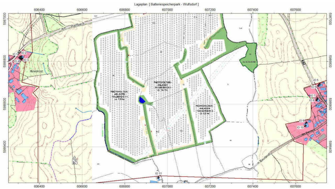
Abbildung 2 Lageplan der maßgeblichen Immissionsorte
