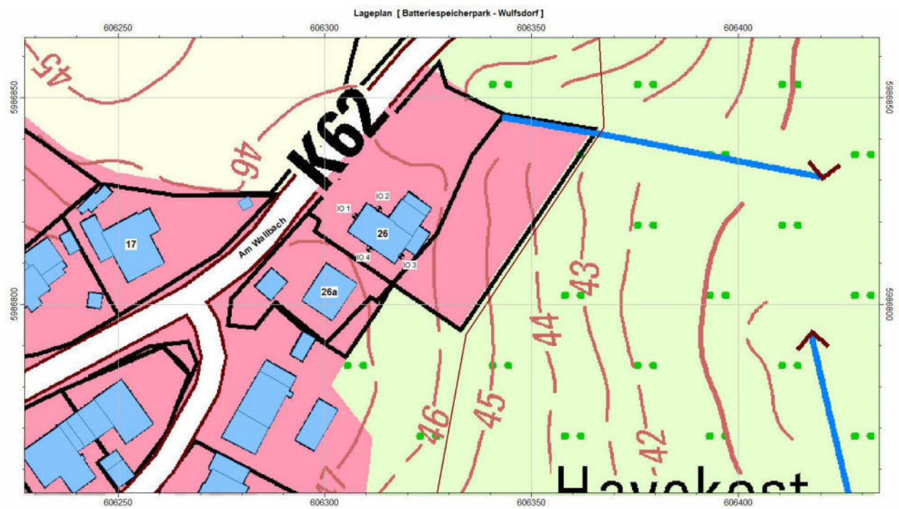
Abbildung 3 Lageplan der maßgeblichen Immissionsorte, Havelkost
