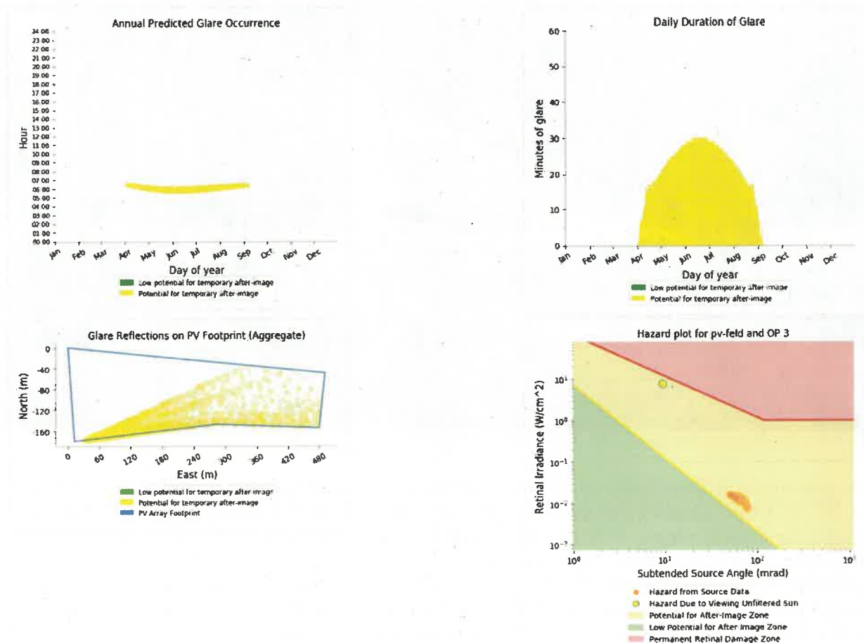
Bild 4.4.3: Ergebnisdetails für Messpunkt P4 (Quelle: Simulationsergebnisse)
