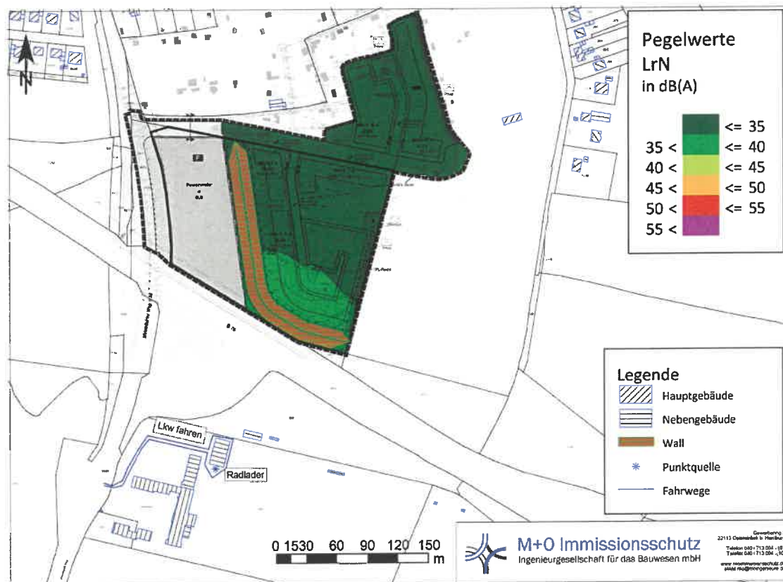
Abbildung 12: Immissionen aus Bauhof (5,6 m über Gelände) nachts
