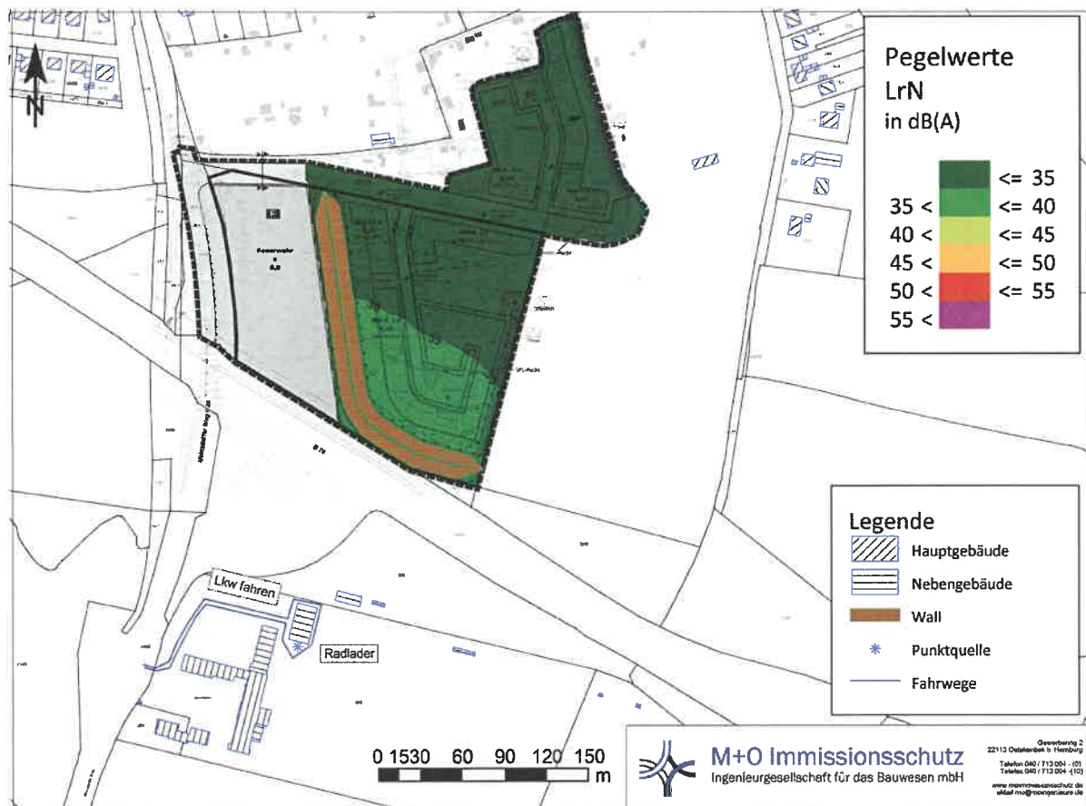
Abbildung 13: Immissionen aus Bauhof (8,4 m über Gelände) nachts
