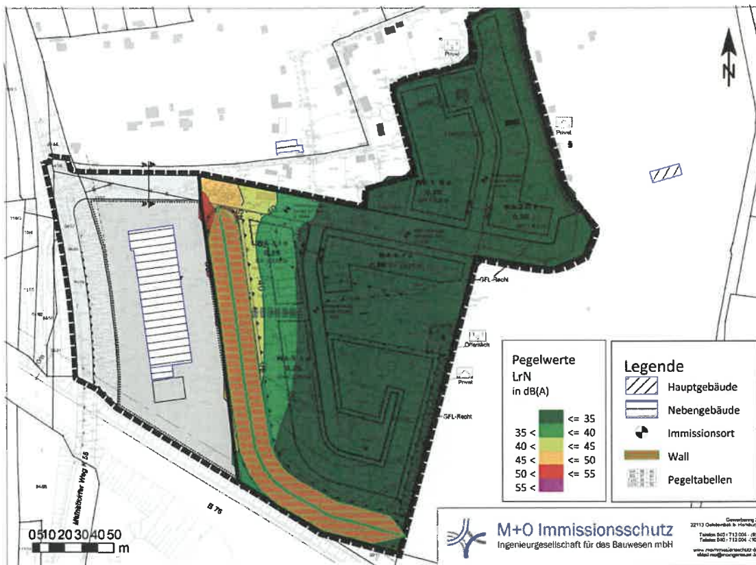
Abbildung 22: Immissionen aus FF Eutin (8,4 m über Gelände) nachts, Übungen
