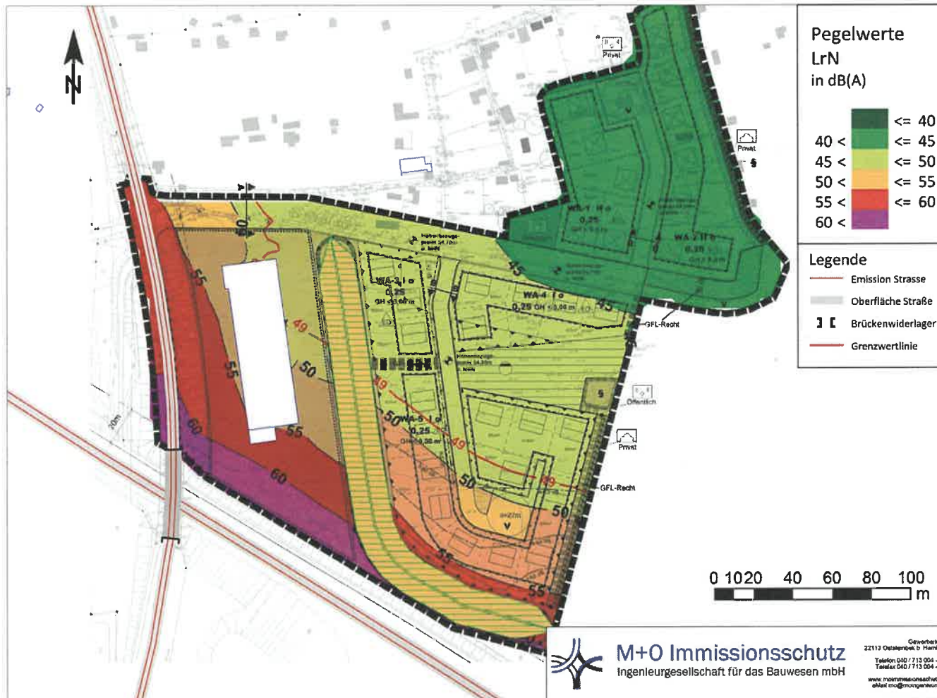
Abbildung 9: Immissionen aus Straßenverkehr (8,4 m über Gelände) nachts
