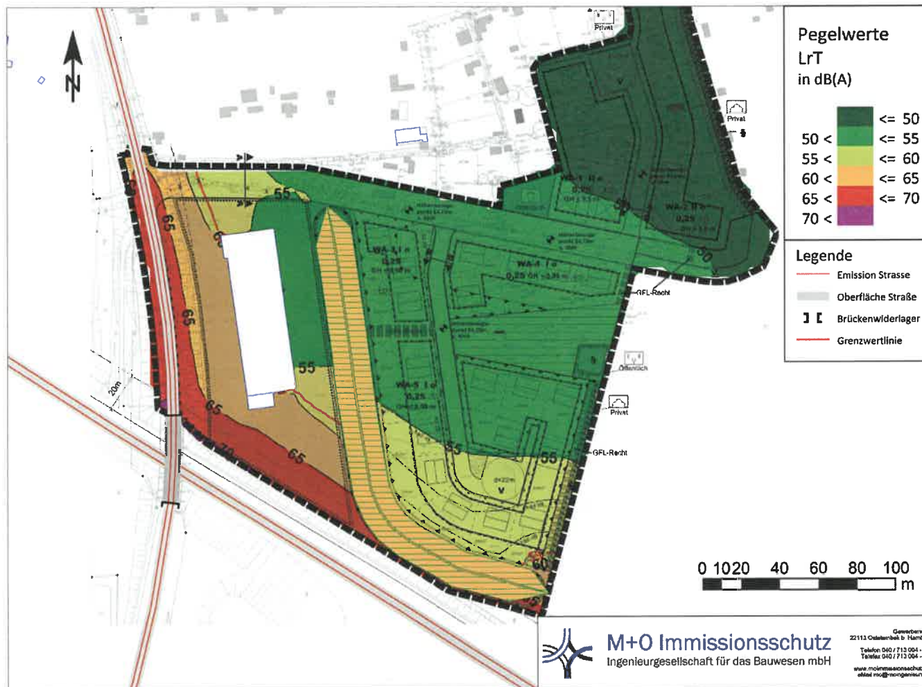
Abbildung 5: Immissionen aus Straßenverkehr (5,6 m über Gelände) tags
