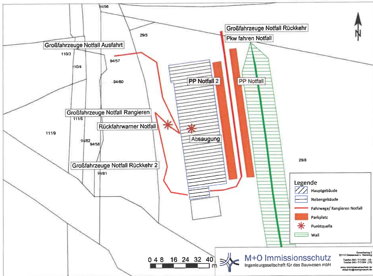
Abbildung 15: Quellplan der FF Eutin Notfall-Einsatz
