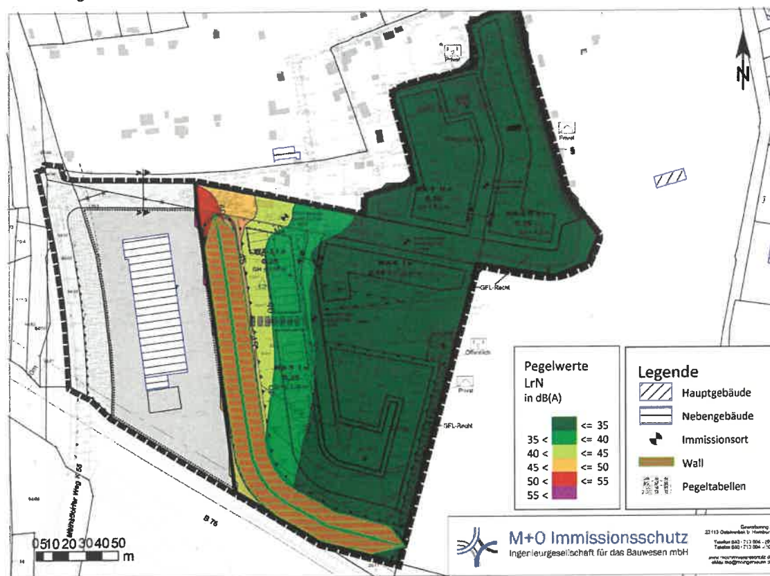
Abbildung 25: Immissionen aus FF Eutin (8,4 m über Gelände) nachts, Notfall-E.
