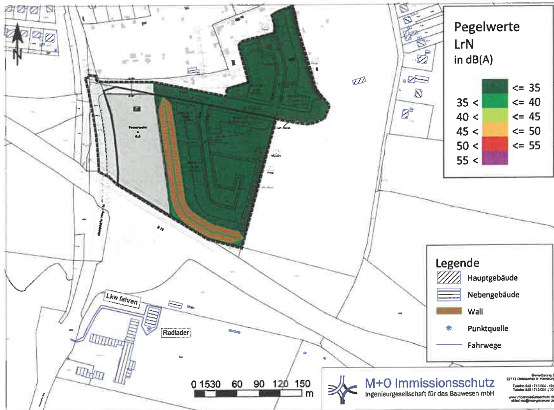
Abbildung 12: Immissionen aus Bauhof (5,6 m über Gelände) nachts
