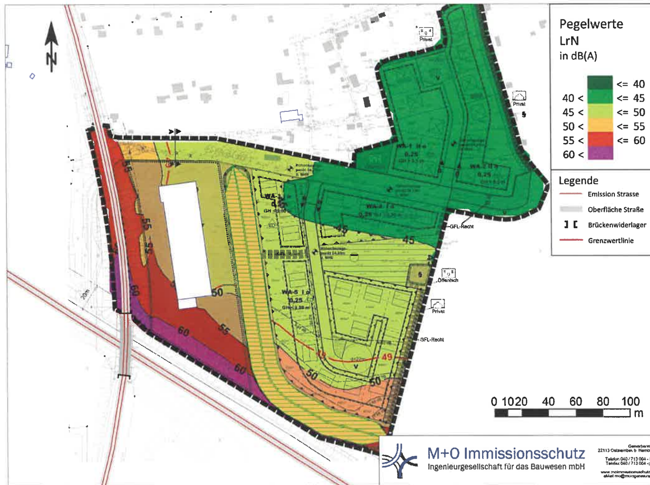
Abbildung 8: Immissionen aus Straßenverkehr (5,6 m über Gelände) nachts
