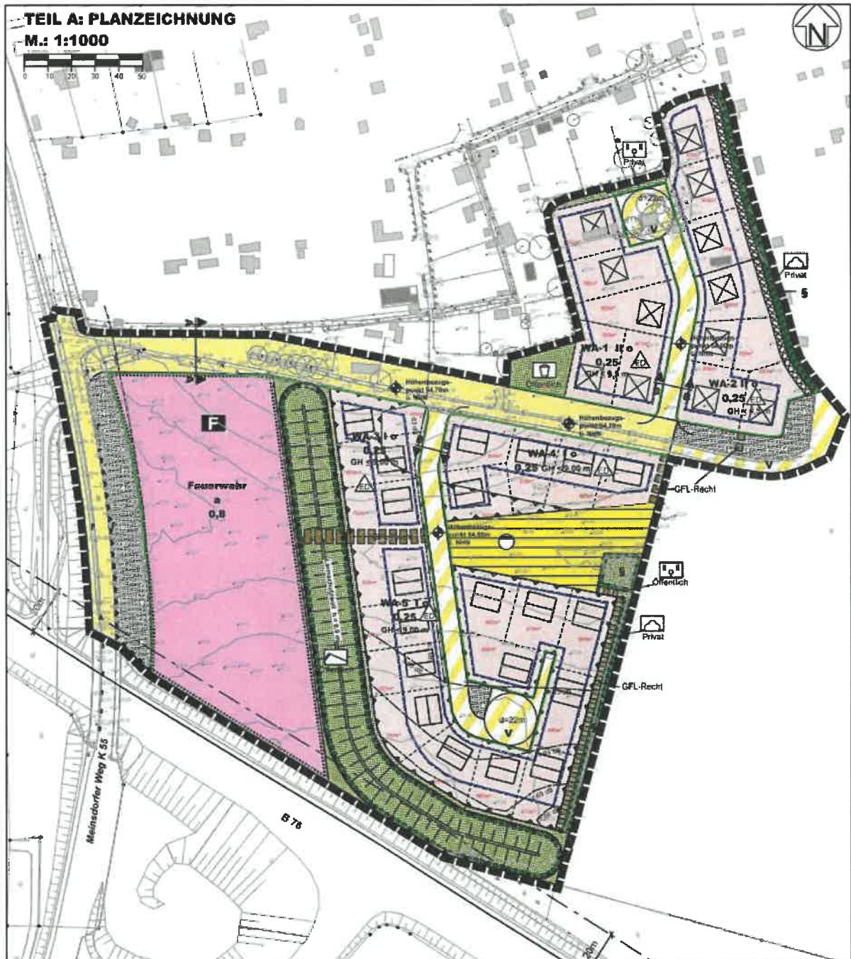
Abbildung 2: Auszug aus dem Vorentwurf zum Bebauungsplan Nr. 143
