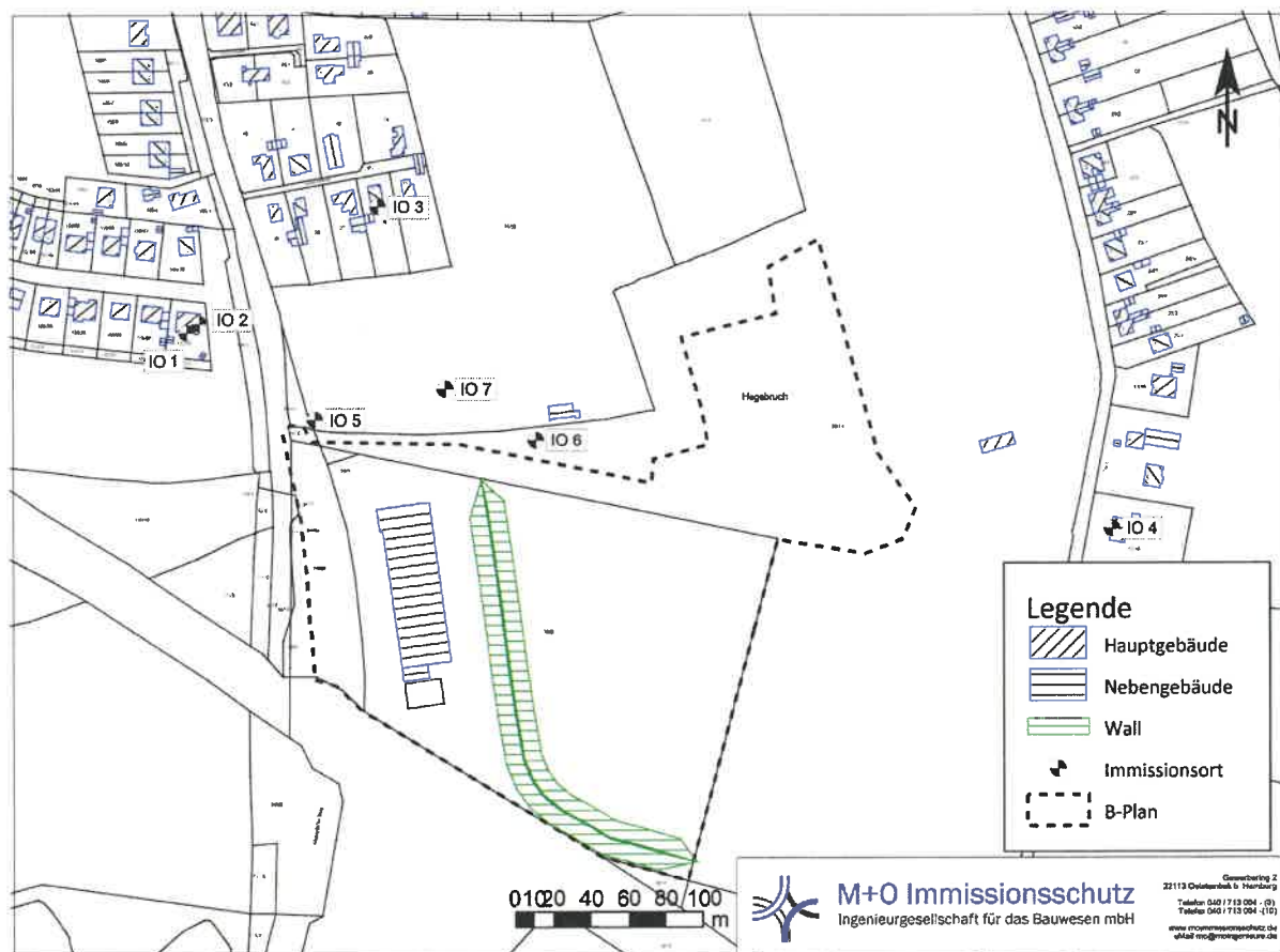
Abbildung 16: Lageplan der Immissionsorte
