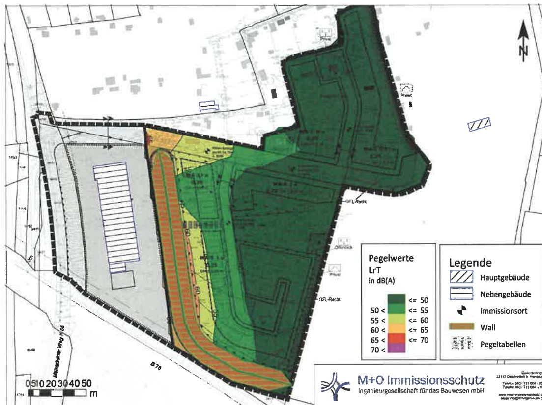
Abbildung 19: Immissionen aus FF Eutin (8,4 m über Gelände) tags, Übungen
