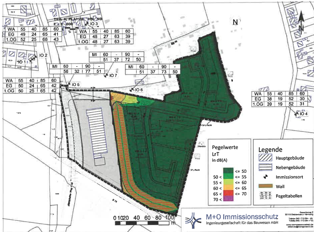
Abbildung 17: Immissionen aus FF Eutin (2,0 m über Gelände) tags, Übungen
