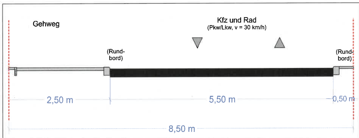
Bild 8-2: Straßenquerschnitt Wohnstraße, Konzeptskizze
