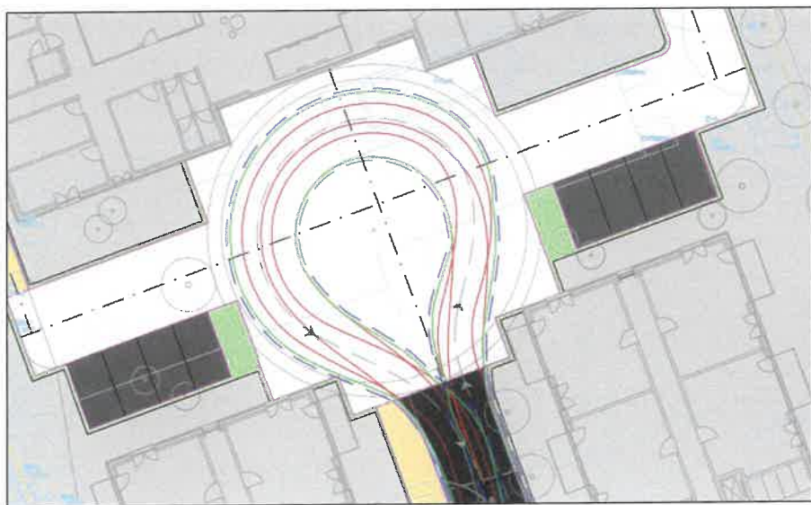
Bild 8-1: Schleppkurve dreiachsiges Müllfahrzeug
