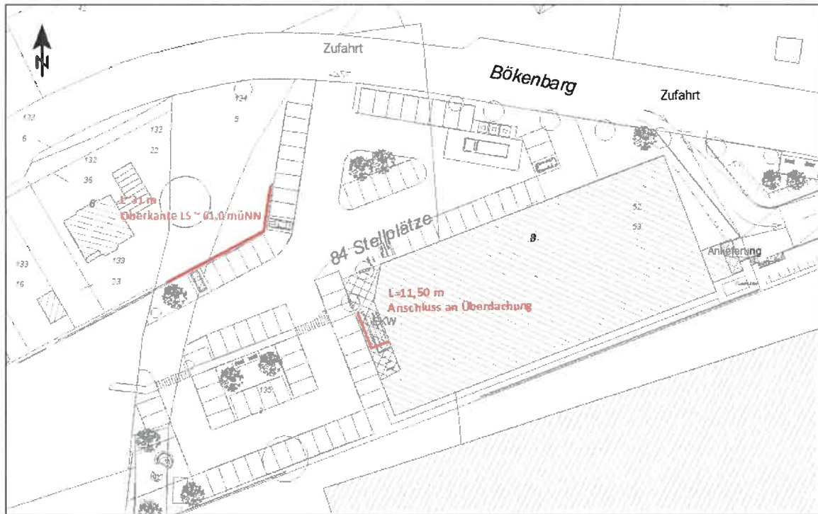
Bild 5.1: Erforderliche Abschirmungen
